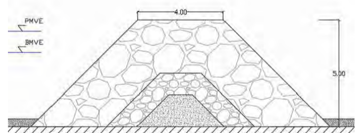
Sección en morro Espigón 3
