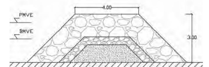
Sección en morro Espigón 3
