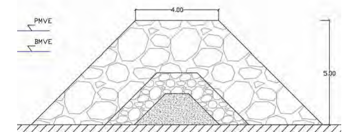
Sección en morro Espigón 2
