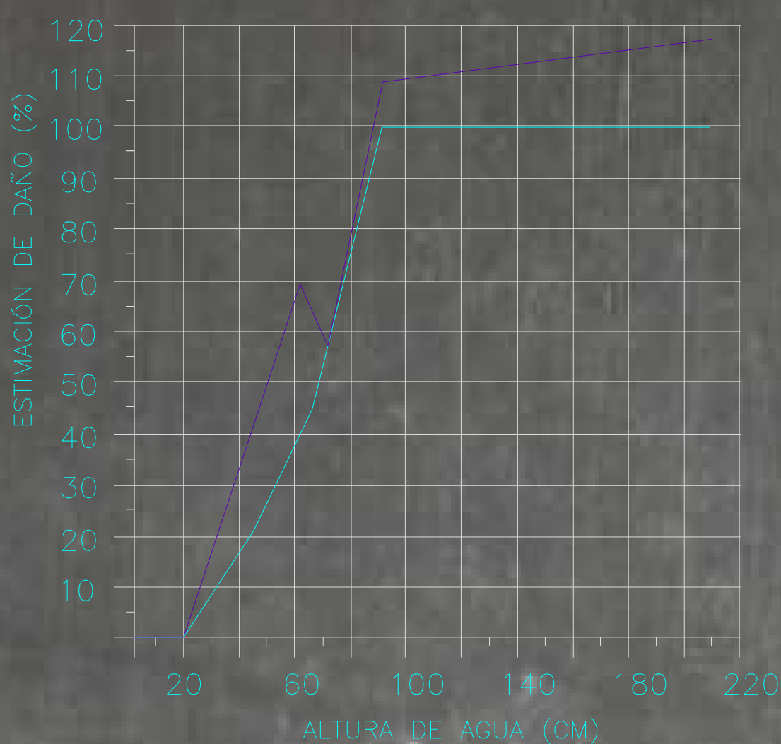
DAÑO SEGÚN ALTURA DE LÁMINA EN INUNDACIÓN EN TÉRMINOS RELATIVOS
